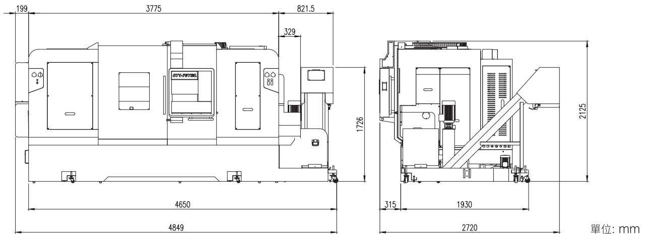
機台外觀尺寸圖
